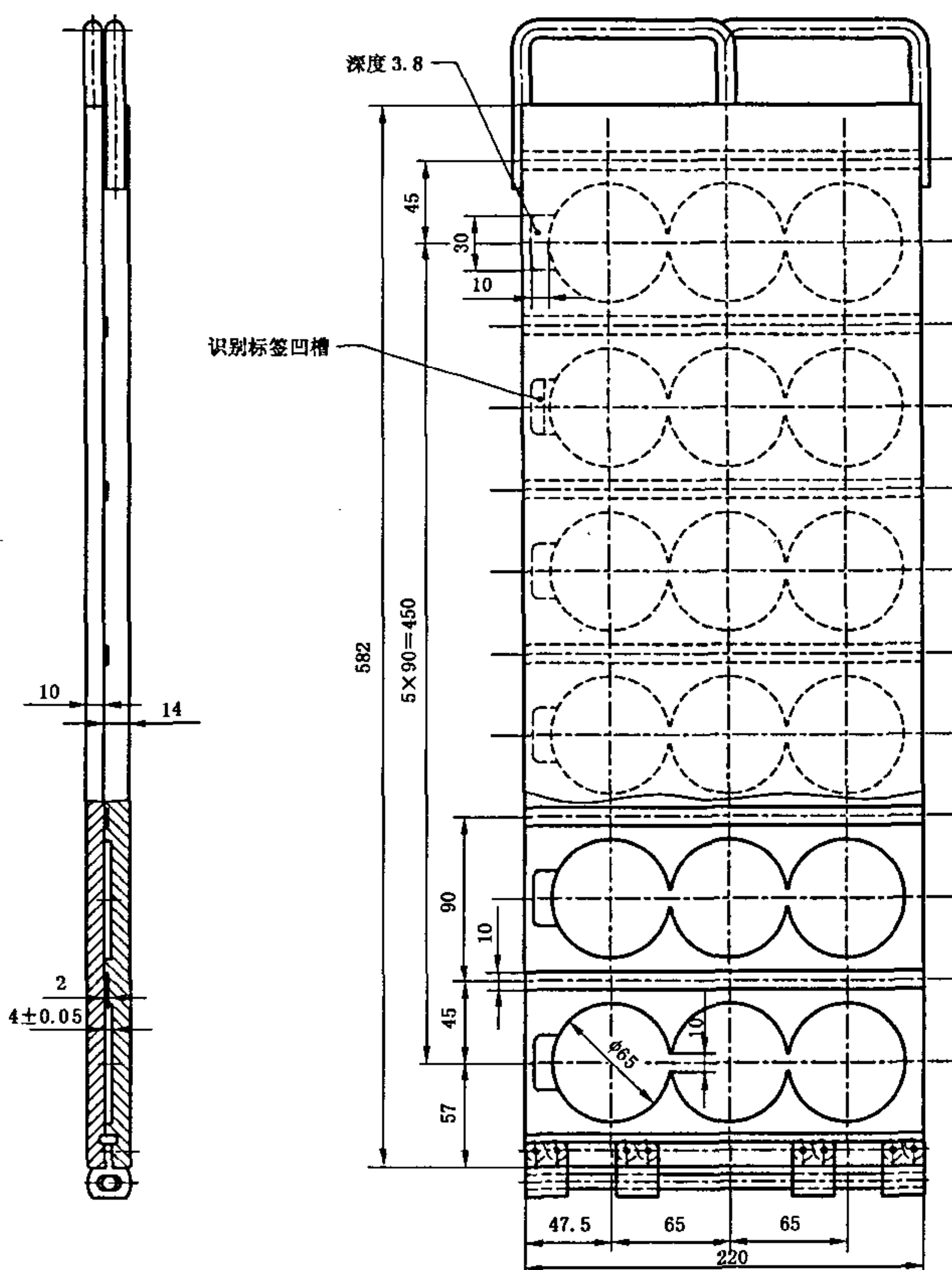
图 2 环状试样圆形硫化胶片模具图
