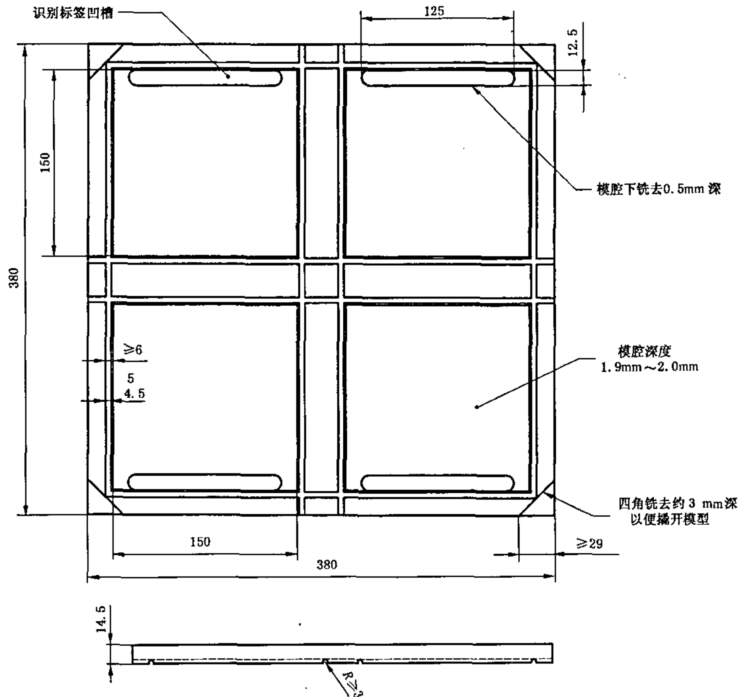
图 1 四腔模具图
